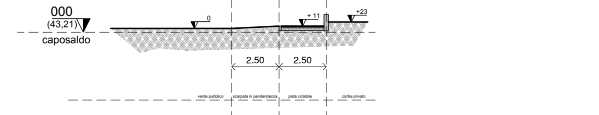
SEZIONE scala 1: 200
