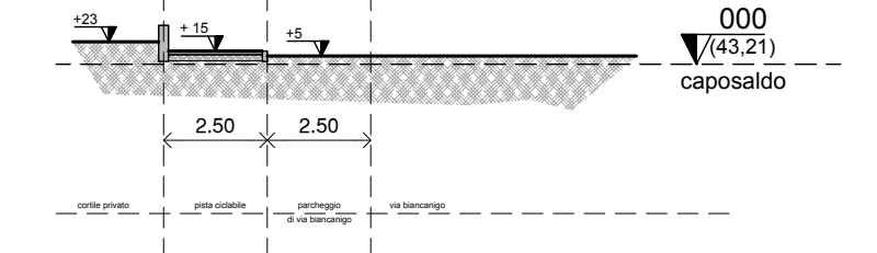
SEZIONE scala 1: 200
